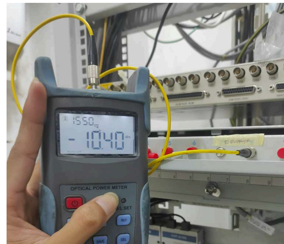
Pengukuran Daya/Redaman Fiber Optik
